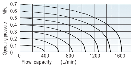
Model: 3L310-10
